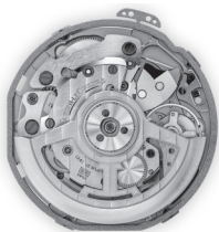
Jaeger-LeCoultre 积家 956 型机芯
